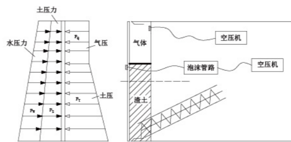
气土联合平衡盾构掘进原理图
